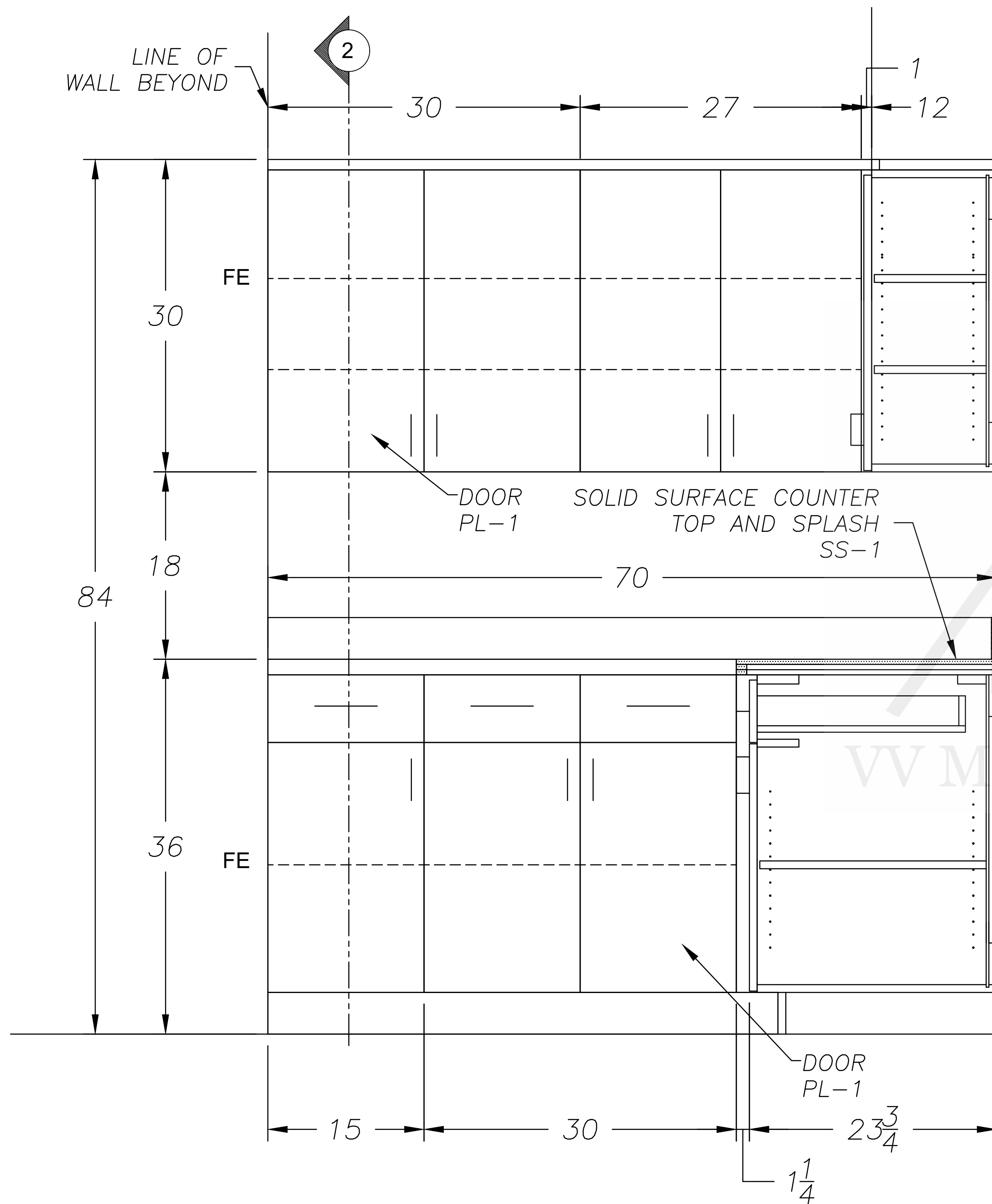
ELEVATION 2 SCALE: 3/4"=1'0"
