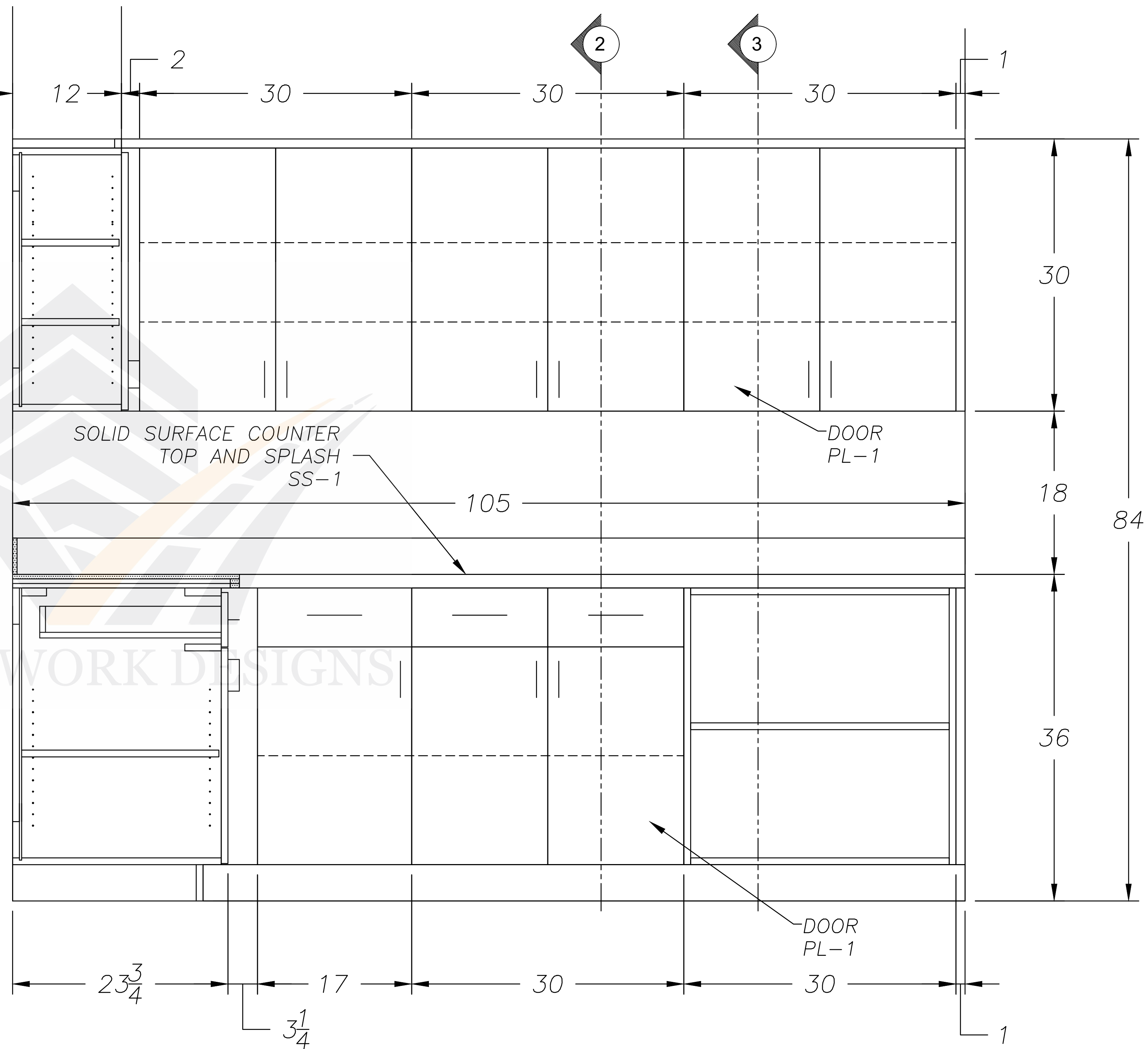
ELEVATION 3 SCALE: 3/4"=1'0"
